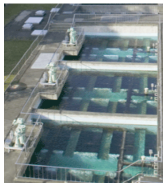
～丸山浄水場ろ過池全景～
