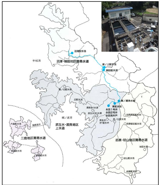
1. 郷ノ浦浄水場～水道施設概略図～
